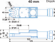
MANYETİK ANAHTAR KAFALARI Düşük Titreşimli Kavrama
